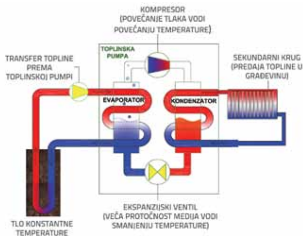
Slika 3. Princip rada geotermalne dizalice topline
