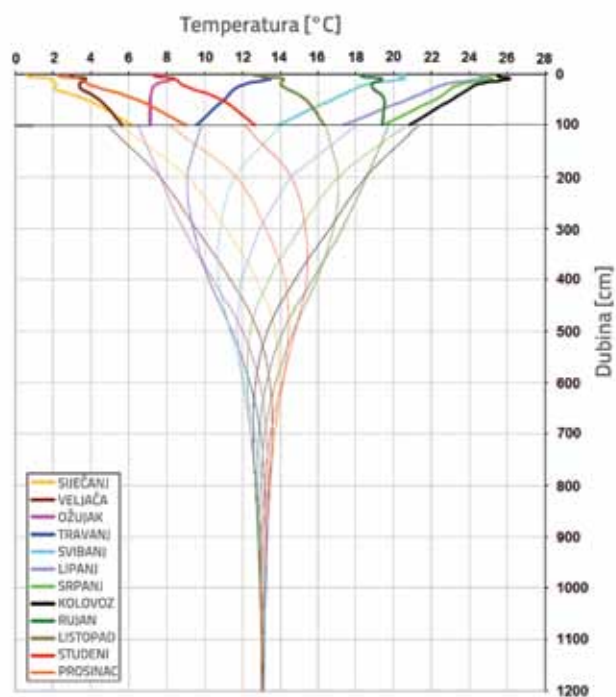
Slika 2. Krivulje promjene temperature po dubini na području grada Zagreba [9]
