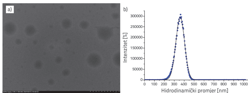
Slika 2. a) TEM mikrograf; b) DLS krivulja nanokompozita CHT/HS
