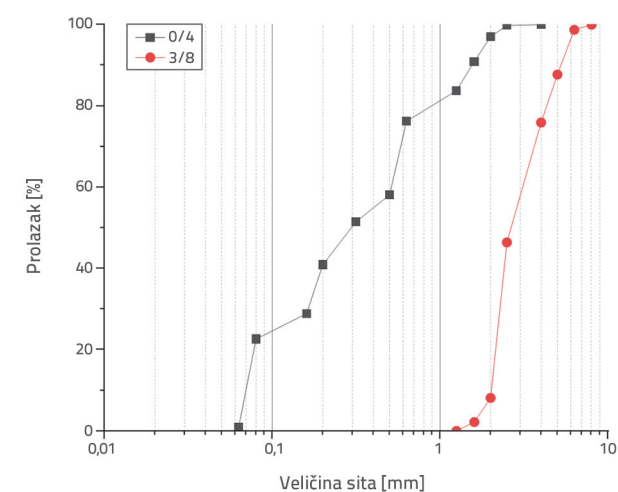
Slika 1. Granulometrijski sastav krupnog i sitnog agregata
