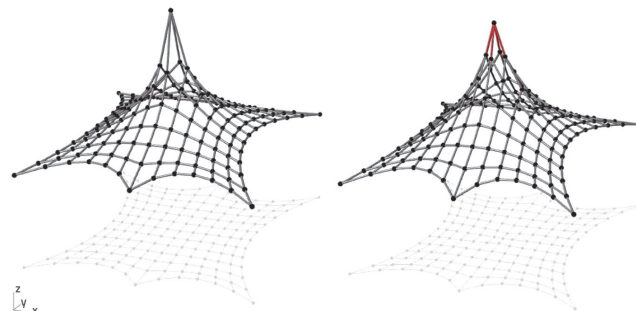
Slika 25. Ravnotežni položaj za zadane gustoće sile i dodatno za zadana ograničenja duljina elemenata oko visoke ležajne točke – model 2.
