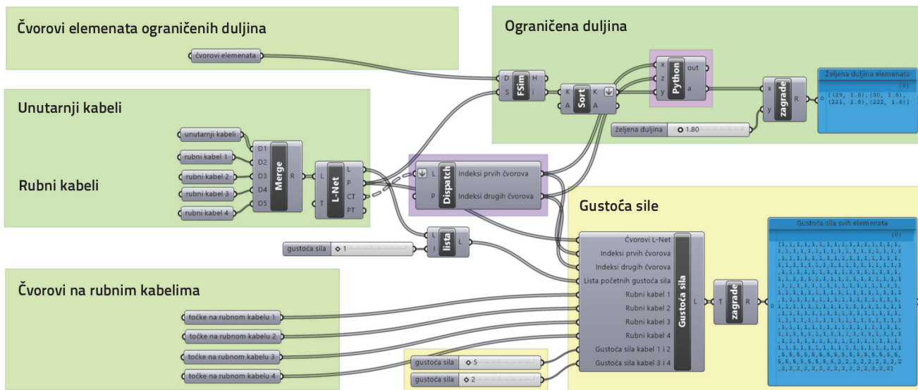
Slika 22. Skripta GH za zadavanje različitih vrijednosti gustoća sile rubnih kabela i ograničenja duljina elemenata
