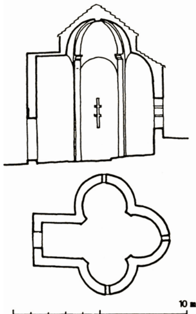
Presjek i tlocrt crkve Sv. Krševana
