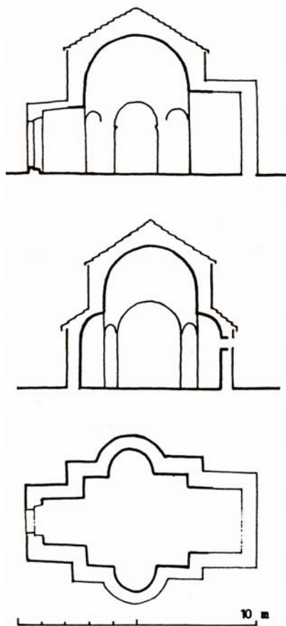
Uzdužni presjek (gore), poprečni presjek (srednja) i tlocrt crkve Sv. Dunata
