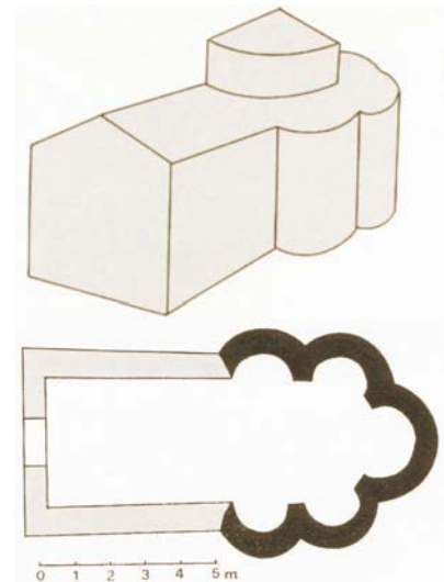
Rekonstrukcija izgleda i tlocrta najstarije crkve Sv. Marije u Škabrnji
