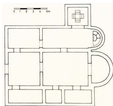
Rekonstrukcija tlocrta starokršćanske crkve u Polači
