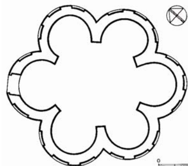
Tlocrt predromaničke šesteroapsidne crkve na Mastirinama u Kašiću
