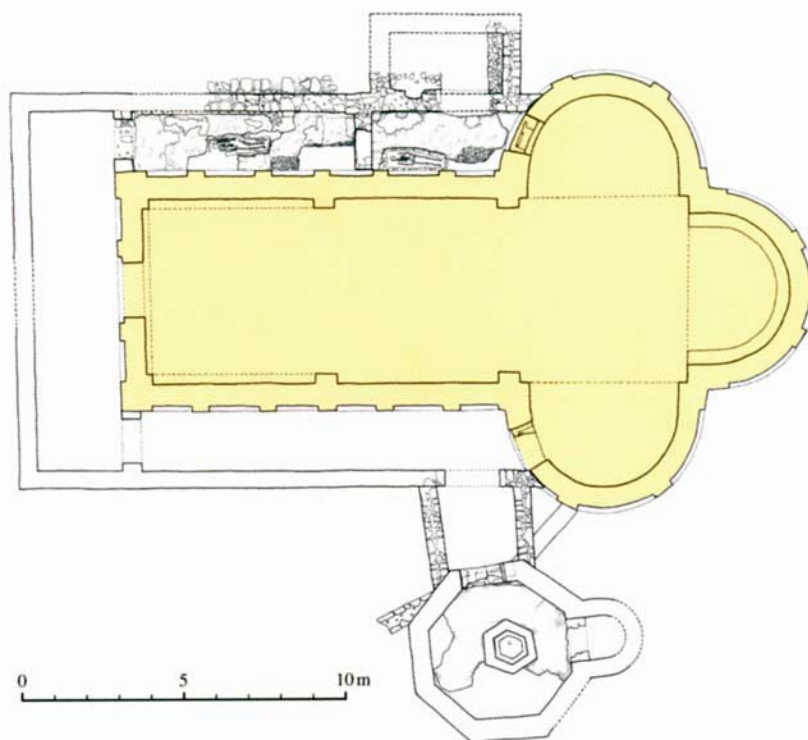
Tlocrt istraženih ostataka starokršćanske crkve Sv. Martina u Pidrasi
