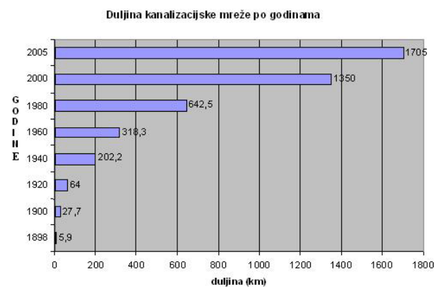
Slika 2. Kronologija izgradnje kanalizacijske mreže grada Zagreba
