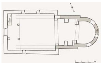
Tlocrt crkve Sv. Stjepana u Stipanskoj luci u Pučišćima
