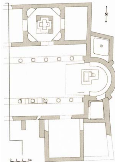
Tlocrt ruševina starokršćanske crkve Sv. Ivana u Postirama
