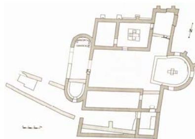
Tlocrt starokršćanske crkve u Lovrečini
