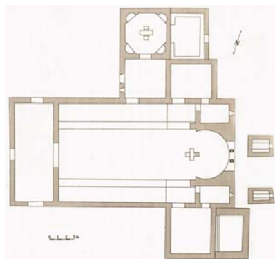
Tlocrt starokršćanske crkve Sv. Ivana Krstitelja u Povljima
