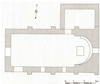
Tlocrt starokršćanske crkve Sv. Jadre između Splitske i Škripa
