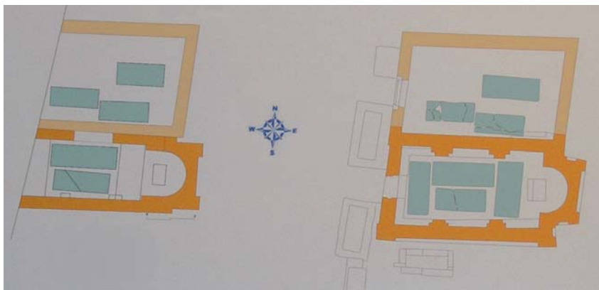
Tlocrt crkve Sv. Mihajla prije i nakon istražnih radova
