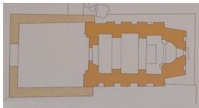
Tlocrt Sv. Nikole prije rekonstrukcije
