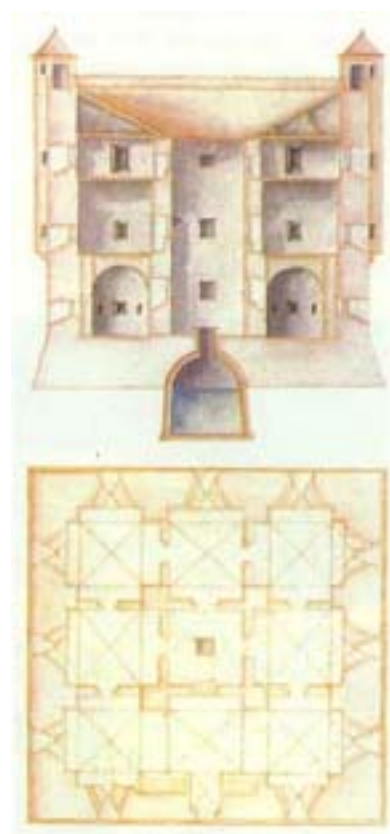
Tlocrt i presjek tvrđave Nehaj Martina Stiera 1660. godine
