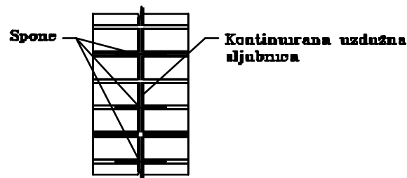
Slika 9. Presjek kroz dvostruki zid bez šupljine između dva sloja
