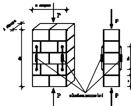
Slika 4. Mali uzorci ziđa (ispitivanja je tlačne čvrstoće)
